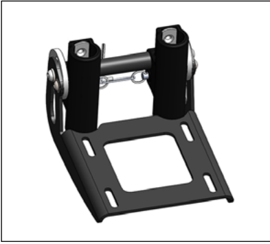
Fußbretthalter mit einstellbarem Winkel, hochklappbar
