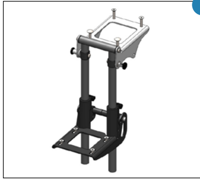
Kniewinkelanlage 90°
