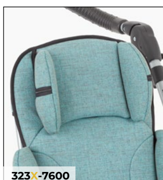
Kopfstützpelotten, niedrige Form
