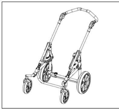
Lenkräder-Vorsatz, für Zusatzgeräte
