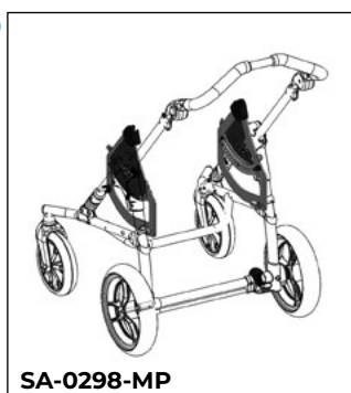
Erhöhung Sitzaufnahme um 10 cm
