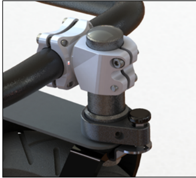
Lenkstopp für Mittellenrad
