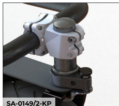
Lenkstopp für Mittlenkgrad
