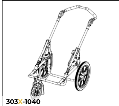
Cross mit Mittellenkrad-Vorsatz, für Zusatzgeräte
