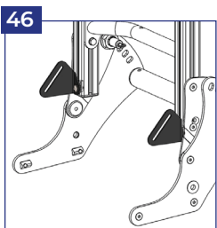
Beckengurtführungen
