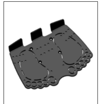
Alu-Fußbrett „footprint“ mit Fersenkante
