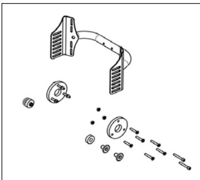
Verbreiterungssatz um 2 cm
