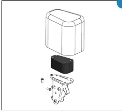
A-Keil Erhöhung um 30 mm
