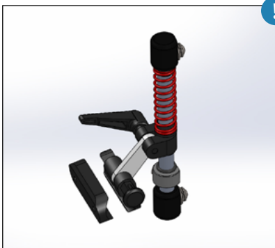
Dynamik Paket für die Rückenbasis „winkelverstellbar“
