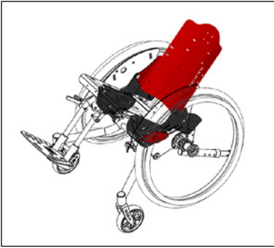
CLEO mit 45° Sitzkantellung, mit winkelverstellbarem & abklappbarem Rücken
