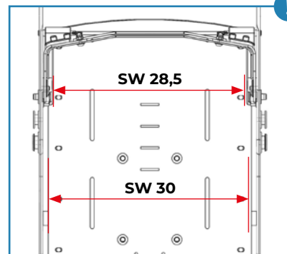
Push bar „wide“, detachable
